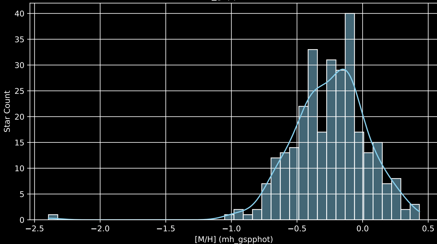
GALAH DR4 Field: [1316] [M/H] (mh_gspphot) (n= 290)
