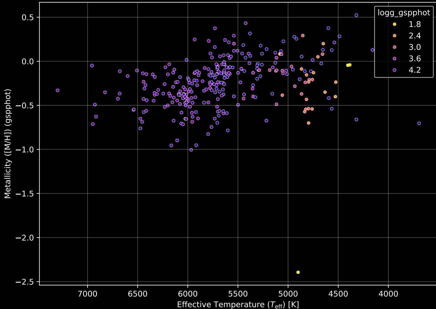
GALAH DR4 Field: [1316] Stellar Population Parameters (n= 291)
