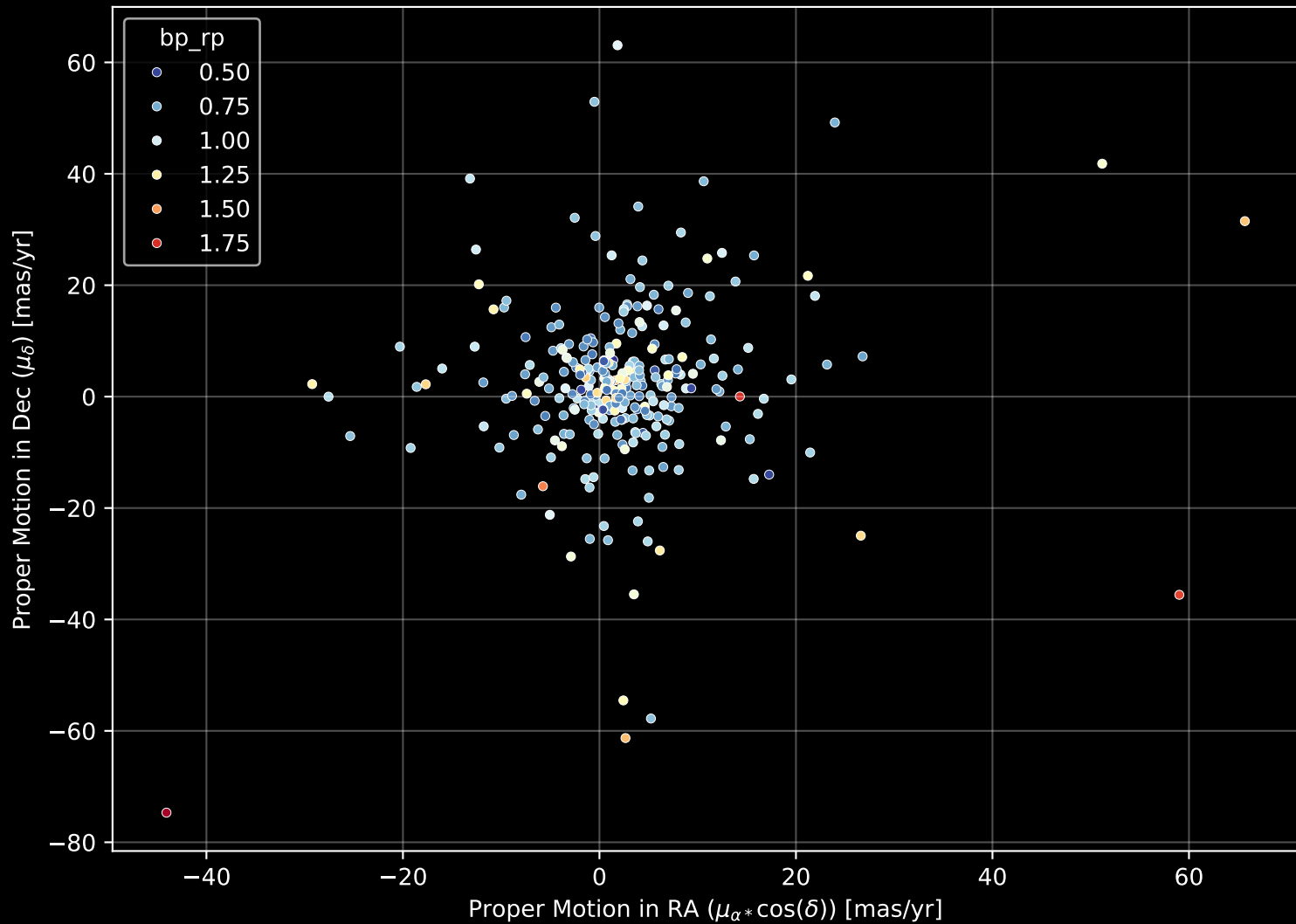
GALAH DR4 Field: [1316] Proper Motion Diagram (n= 291)
