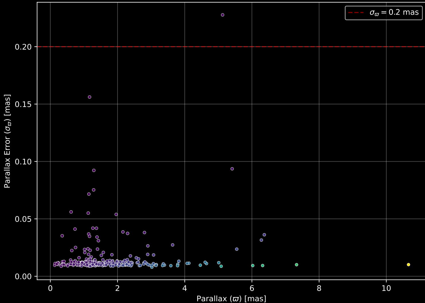
GALAH DR4 Field: [1316] Parallax Quality (n= 291)
